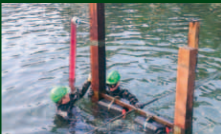
Duikers spuiten de palen m.b.v. JCB200
